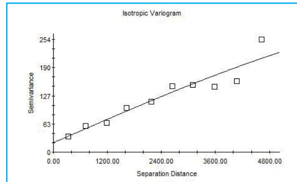
شکل ۵. تغییرنگار تجربی در عمق ۰-۱۵ cm برای دو فلز آرسنیک و کروم
