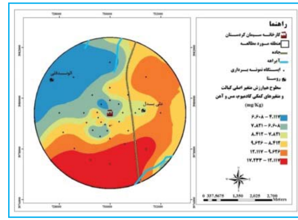
(Co)
