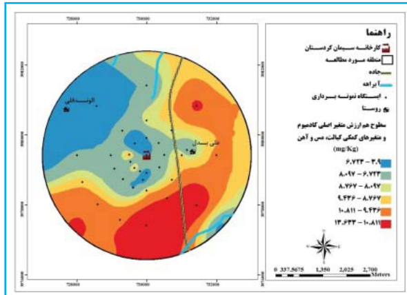
(Cd)
