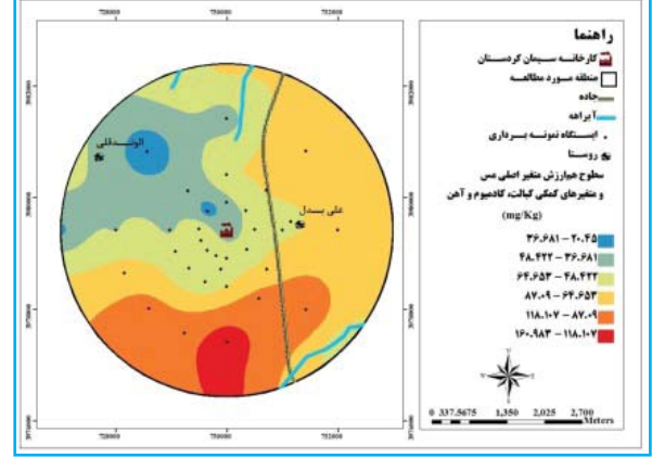
(Cu)
