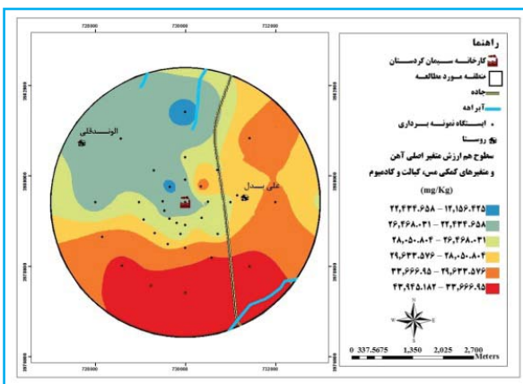
(Fe)
