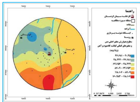
(Cu)
