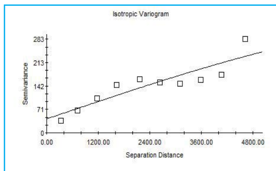
(Cr)
