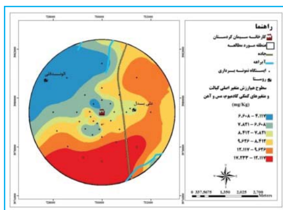
(Co)
