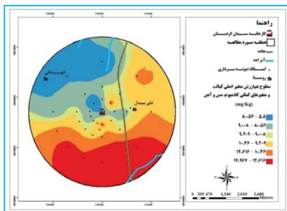
(Co)
