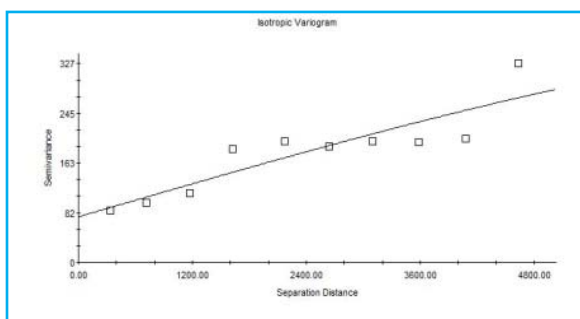
(Cr)
