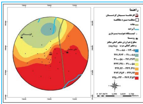
(Mn)
