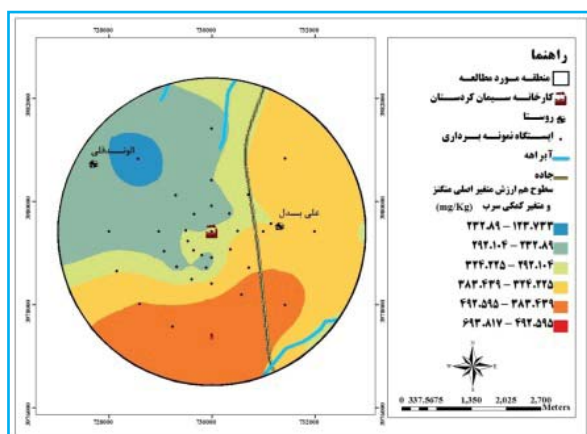
(Mn)
