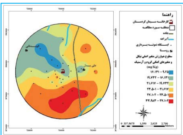
(Ni)
