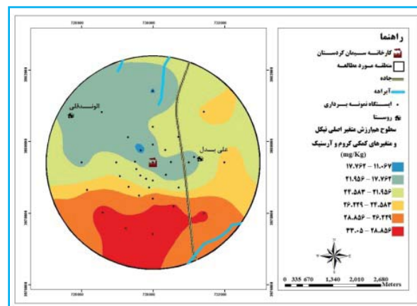
(Ni)
