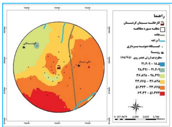
(Zn)
