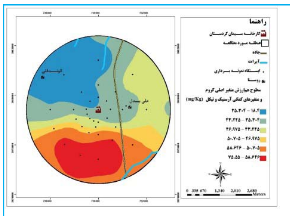
(Cr)
