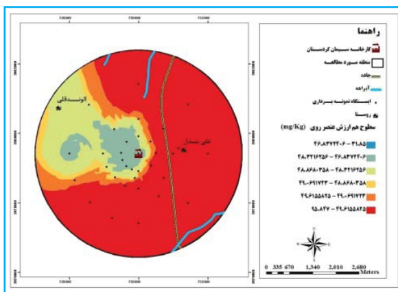
(Zn)
