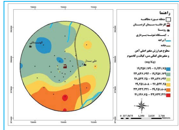
(Fe)
