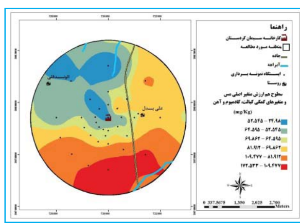
(Cu)
