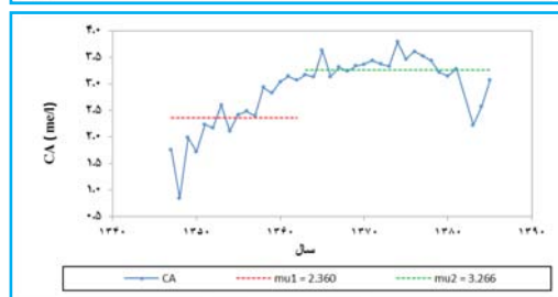
شکل ۲. روند تغییرات پارامترهای \text{pH} ، \text{EC} ، \text{HCO}_3^- ، \text{CL} ، \text{SO}_4^{2-} ، \text{Ca} ، \text{Mg} ، \text{Na} و \text{SAR} در ایستگاه قورباغستان
