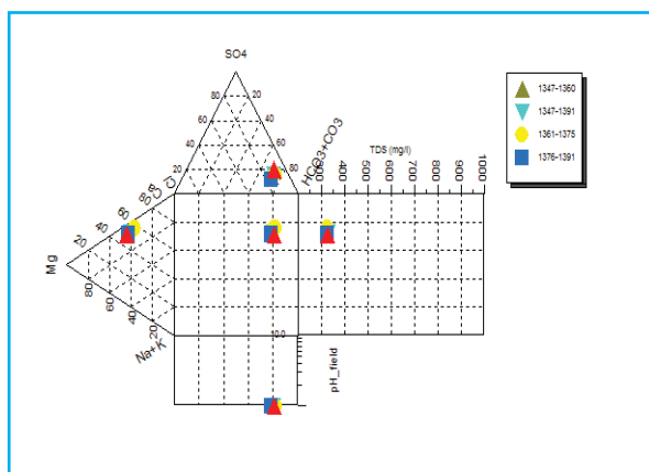
شکل ۵. نمودار دورو مربوط به ایستگاه‌های قورباغستان (راست) و دوآب مرک (چپ)
