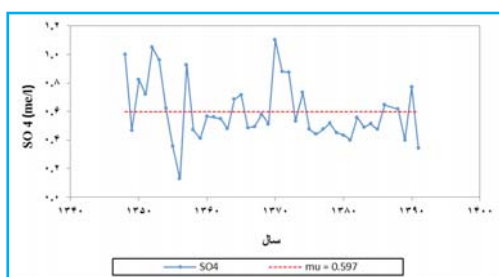
شکل ۳. روند تغییرات پارامترهای pH، EC، \text{HCO}_3^- ، \text{CL} ، \text{SO}_4 ، \text{Ca} ، \text{Mg} ، \text{Na} و SAR در ایستگاه دوآب مرگ
