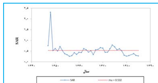
ادامه شکل ۲. روند تغییرات پارامترهای pH، EC، \text{HCO}_3^- ، \text{CL} ، \text{SO}_4 ، \text{Ca} ، \text{Mg} ، \text{Na} و SAR در ایستگاه قورباغستان
