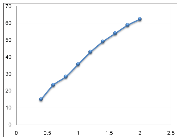
نمودار ۳: کارایی حذف فلوراید در غلظت‌های مختلف جاذب در pH بهینه ۷ و زمان تماس بهینه ۶۰ دقیقه
