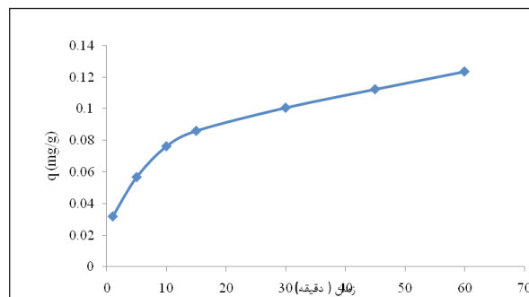
نمودار ۴: ظرفیت جذب بر زمان در غلظت جاذب ۲ میلی گرم بر لیتر و غلظت فلوراید ۴ میلی گرم بر لیتر
