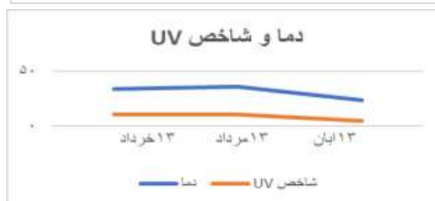
نمودار ۲. بارش و آفتابی، دما و شاخص UV
