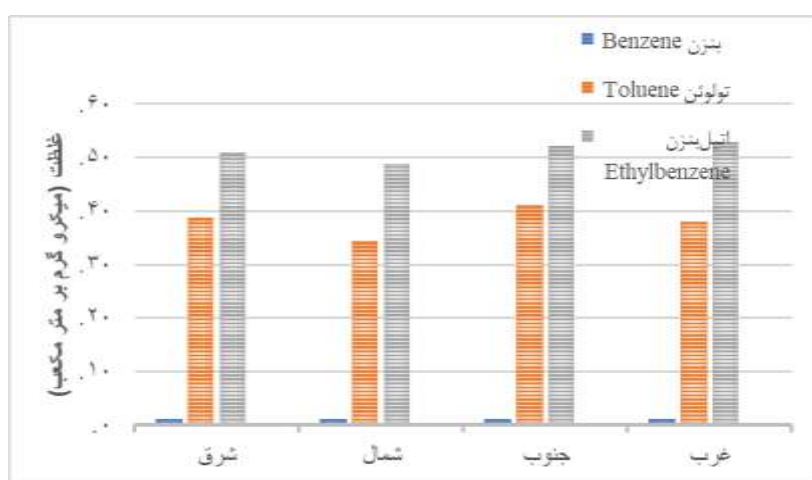
نمودار ۱. غلظت ترکیبات BTEX در ایستگاه‌های مختلف جهت جغرافیایی
