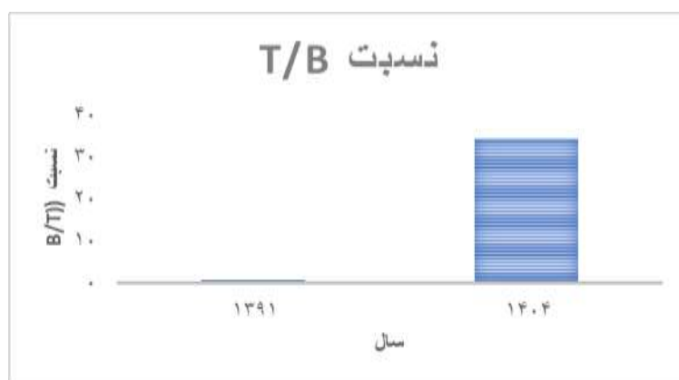
نمودار ۴. نسبت تولوئن به بنزن (T/B) در سال ۱۳۹۱ و ۱۴۰۴
