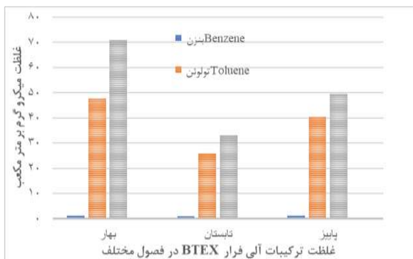
نمودار ۳. تغییرات فصلی میانگین غلظت BTEX در سال ۱۴۰۴
