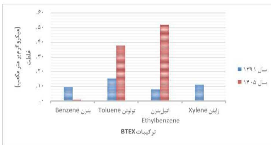
نمودار ۵. مقایسه میانگین غلظت BTEX بین سال‌های ۱۳۹۱ و ۱۴۰۴
