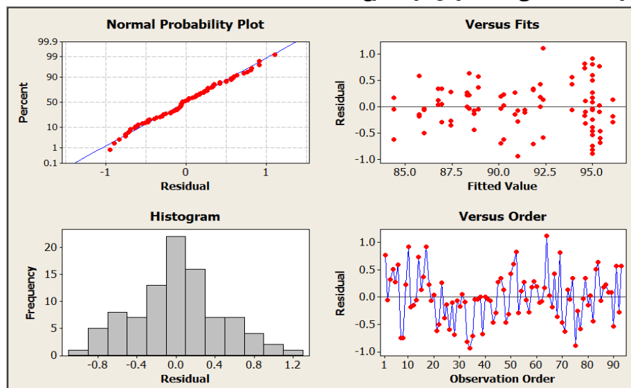
نمودار ۱. بررسی گرافیکی مفروضات مدل آنالیز واریانس در حذف COD در فرآیند سونوکاتالیزستی
