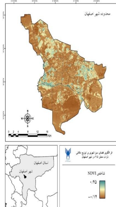
شکل ۳. نقشه پوشش گیاهی تفاضلی نرمال شده تولید شده با استفاده از تصاویر ماهواره لندست برای شهر اصفهان
