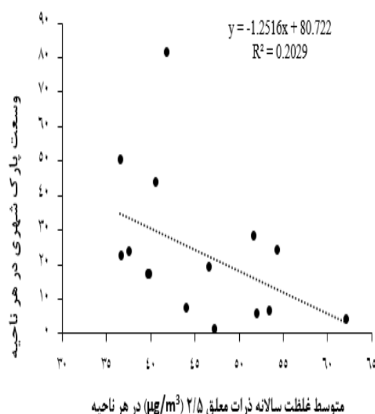
شکل ۶. ارتباط بین غلظت سالانه ذرات معلق ۲/۵ (µg/m³) با وسعت پارک های شهر اصفهان
