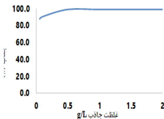
نمودار ۴. بررسی اثر غلظت جاذب بر میزان درصد جذب یون سرب (II) از محلول‌های آبی با استفاده از برگ گیاه نیشکر
