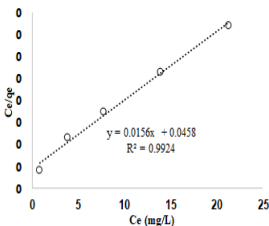
نمودار ۵. مدل ایزوترم لانگمیر جذب یون سرب (II) از محلول‌های آبی با استفاده از برگ گیاه نیشکر
