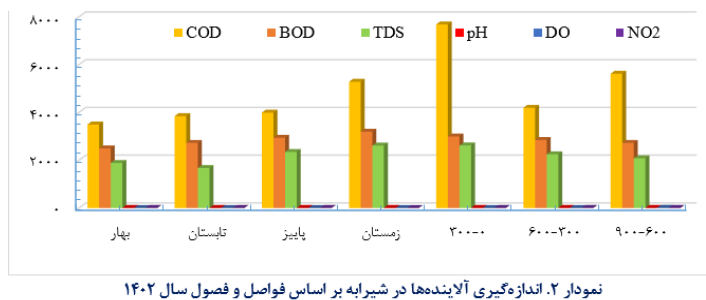
نمودار ۲. اندازه‌گیری آلاینده‌ها در شیرابه بر اساس فواصل و فصول سال ۱۴۰۲
