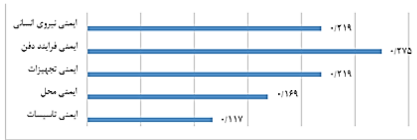
نمودار ۲: وزن هریک از پارامترهای درجه ۱ ایمنی
