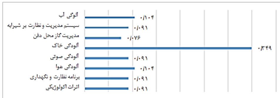
نمودار ۴: وزن هریک از پارامترهای درجه ۱ محیط زیست
