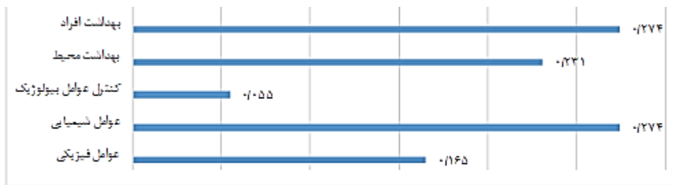
نمودار ۳: وزن هریک از پارامترهای درجه ۱ بهداشت
