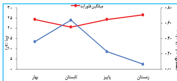
نمودار ۱. تغییرات میانگین غلظت فصلی فلوراید و میانگین دمای فصلی در شهرستان همدان در سال ۱۳۹۸
