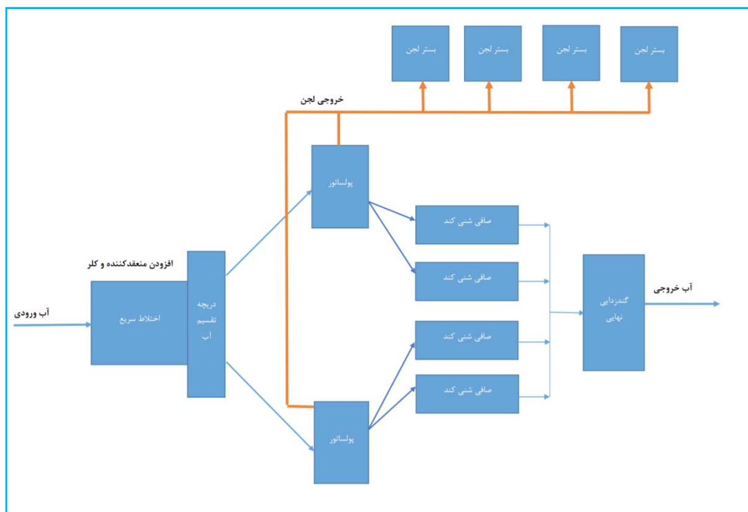
شکل ۱. شماتیک مراحل مختلف تصفیه آب در تصفیه‌خانه آب شهر طبرس
