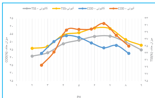
نمودار ۳. تأثیر pH بر میزان حذف COD و TSS توسط کمک منعقدکننده کاتیونی و آنیونی
