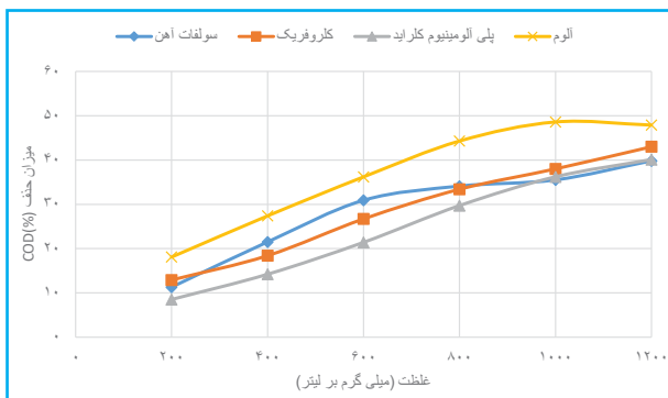
نمودار ۷. تأثیر غلظت ترکیب منعقدکننده و کمک منعقدکننده پلیمری بر میزان حذف COD
