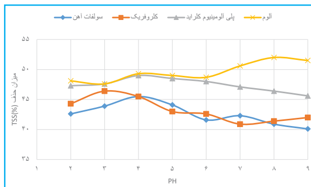
نمودار ۲. تأثیر pH بر میزان حذف TSS
