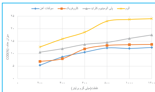
نمودار ۴. تأثیر غلظت ماده منعقدکننده بر میزان حذف COD
