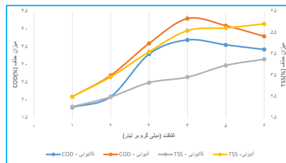
نمودار ۸. تأثیر غلظت کمک منعقدکننده پلیمری بر میزان حذف COD و TSS
