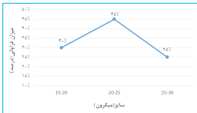
نمودار ۲. سایز ذرات کمتر از ۳۷ میکرون و میزان فراوانی آن
