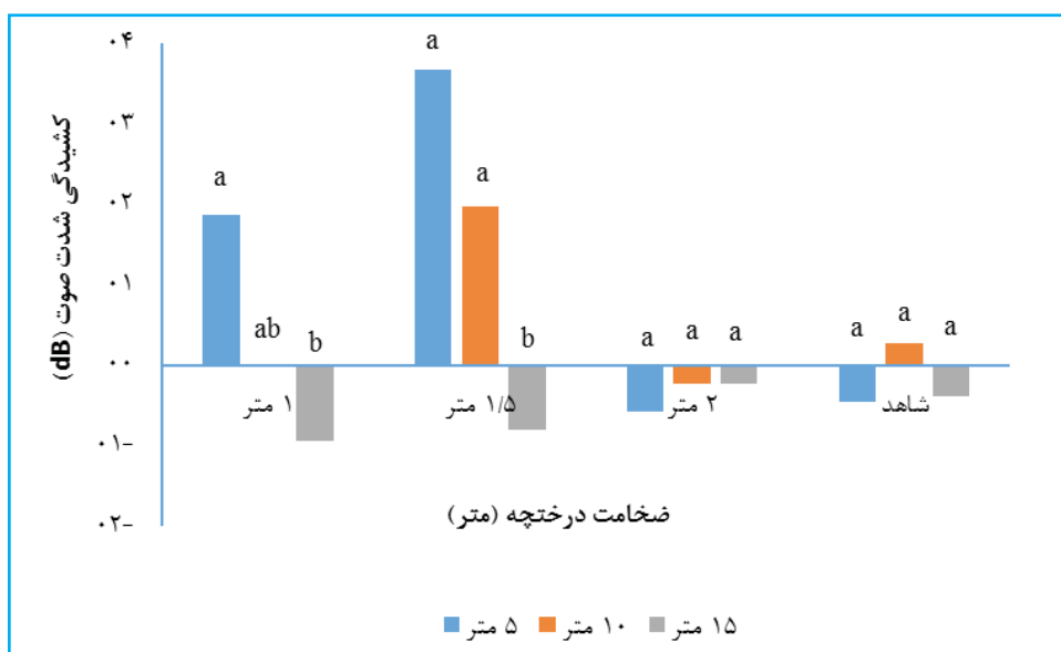
نمودار ۴. اثر برهمکنش فاصله منبع صوت از درختچه و ضخامت درختچه بر کشیدگی شدت صوت (دسی‌بل) * ستون‌هایی با حرف مشابه در سطح احتمال ۵٪ بر اساس آزمون حداقل اختلاف معنی‌دار (LSD)، تفاوت معنی‌داری ندارند.
