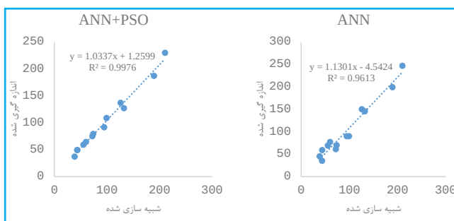
نمودار ۳. نمودار پراکندگی داده‌های اندازه‌گیری و شبیه‌سازی شده سطح آب زیرزمینی بر حسب سانتیمتر
