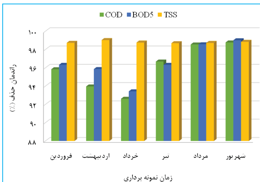
نمودار ۱. راندمان حذف BOD_5 ، COD و TSS در طول دوره ۶ ماهه نمونه برداری
