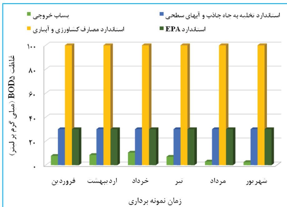
نمودار ۳. مقایسه مقادیر BOD 5 در پساب خروجی تصفیه‌خانه فاضلاب شهر اردکان با استاندارد
