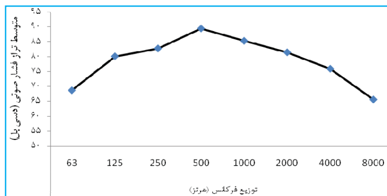
نمودار ۱. متوسط تراز فشار صوت در فرکانس‌های مرکزی اکتاوباند (شبکه توزین فرکانسی C)
