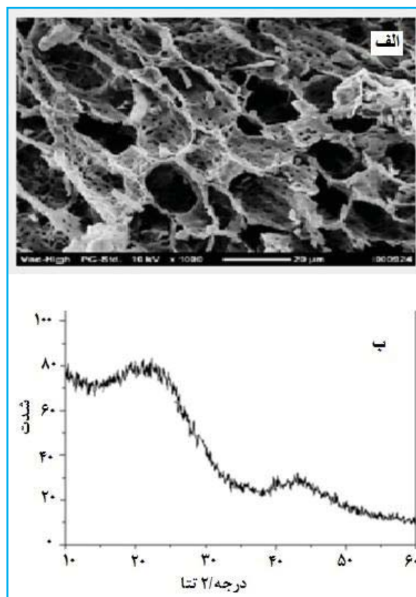
شکل ۱. الف) تصویر میکروسکوپ الکترونی روبشی کرین فعال گرانولی (با بزرگ‌نمایی ۱۰۰۰ برابر)، ب) الگوی پراش اشعه ایکس کرین فعال گرانولی
