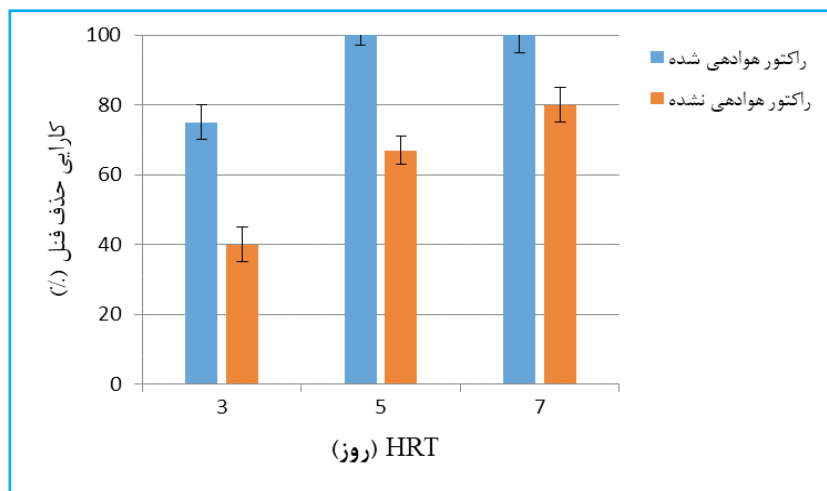
شکل ۲. نمودار راندمان حذف فنل در HRTهای مختلف، غلظت فنل ورودی: ۲۰۰۰ میلی گرم برلیتر
