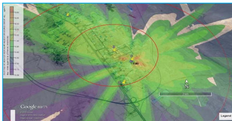
شکل ۲. بیشینه غلظت ساعتی ذرات معلق در فاصله ۲۵۰ متری دودکش نوآوران
