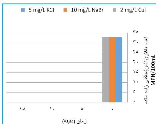
شکل ۲. تعداد باکتری اشريشیاکلی زنده مانده در جریان الکتریکی ۵۰۰ mA توأم با حضور حمایت کننده های الکترولیتی پتاسیم کلراید، سدیم برمید و یدیدمس در ولتاژ ۴/۵ ولت و pH=۷
