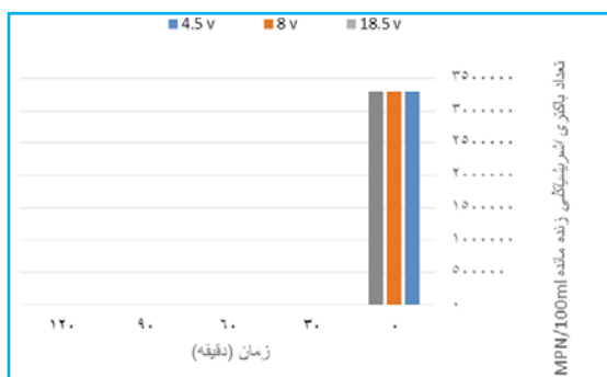
شکل ۴. بررسی تعداد اشريشیاکلی زنده مانده در جریان الکتریکی ۵۰۰ mA در pH=۷ (بدون الکترولیت)
