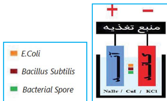
شکل ۱. شمای راکتور مورد استفاده در تحقیق
