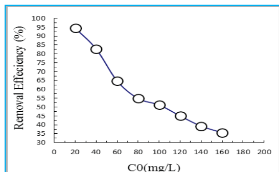
نمودار ۴. بررسی راندمان حذف در غلظت‌های مختلف سولفا دی متوکسین (حجم محلول آنتی‌بیوتیک: ۵۰ mL، مقدار نانولوله g ۰/۰۱، زمان تماس ۶۰ min)
