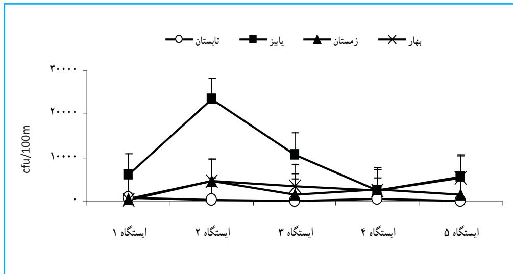
نمودار ۵. تغییرات میانگین کلیفرم کل در فصل‌های مختلف در ایستگاه‌های مختلف سد آزاد سنندج سال ۹۵-۱۳۹۴
