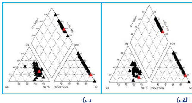
شکل ۳. نمودار پایپر برای ایستگاه‌های: الف) خونیک‌علیا و ب) فرخی
