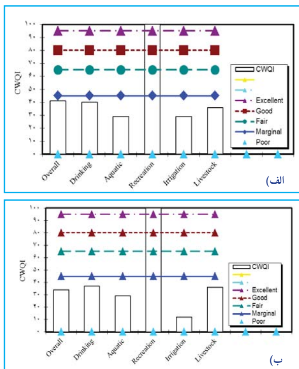
شکل ۲. شرایط کیفی به دست آمده از نرم‌افزار CWQI در ایستگاه‌های: الف) خونیک‌علیا و ب) فرخی
