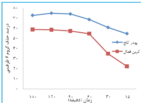
شکل ۲. تأثیر زمان تماس بر روی کارایی حذف (pH=۳) برای پودر و pH=۱ برای کربن فعال آن، مقدار ماده جاذب ۰.۰۰ gr/۲، غلظت اولیه کروم شش ظرفیتی ۵۰ L/mg و دما ۲۲°C)
