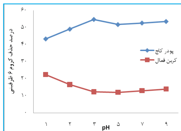
شکل ۴. تأثیر تغییرات pH بر روی کارایی حذف (غلظت اولیه کروم شش ظرفیتی ۵۰ L/mg، مقدار ماده جاذب ۰.۰۰ gr/۲، زمان تماس ۱۵ min و دما ۲۲°C)
