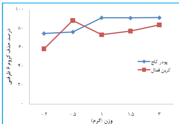
شکل ۳. اثر وزن جاذب در راندمان حذف کروم شش ظرفیتی (pH=۳) برای پودر و pH=۱ برای کربن فعال آن، غلظت اولیه کروم ۵۰ L/mg، زمان تماس ۱۲۰ min و دما ۲۲°C)
